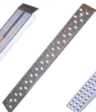
51.525 Uppkörningsramp för Mc, Gräsklippare Längd: 1.6 m Bredd: 20 cm Maxlast/St 250 Kg
