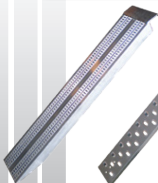
51.524 Uppkörningsramp för Bobcat Längd: 1.55 m Bredd: 30 cm Maxlast/Par 3,5 ton
